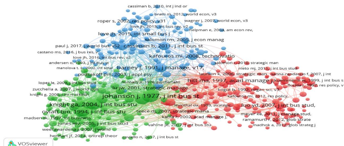
Figura 5 – Mapa de Cocitação
