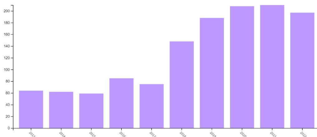
Figura 2 – Evolução das Publicações sobre Inovação e Internacionalização de Empresas na Web of Science.
