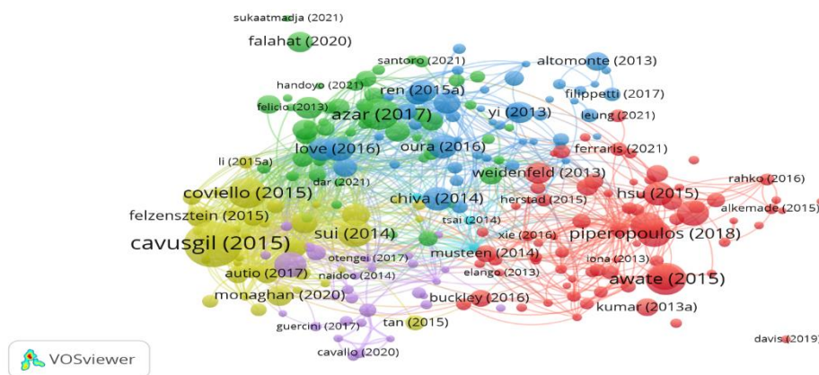
Figura 6 – Mapa de Pareamento Bibliográfico
