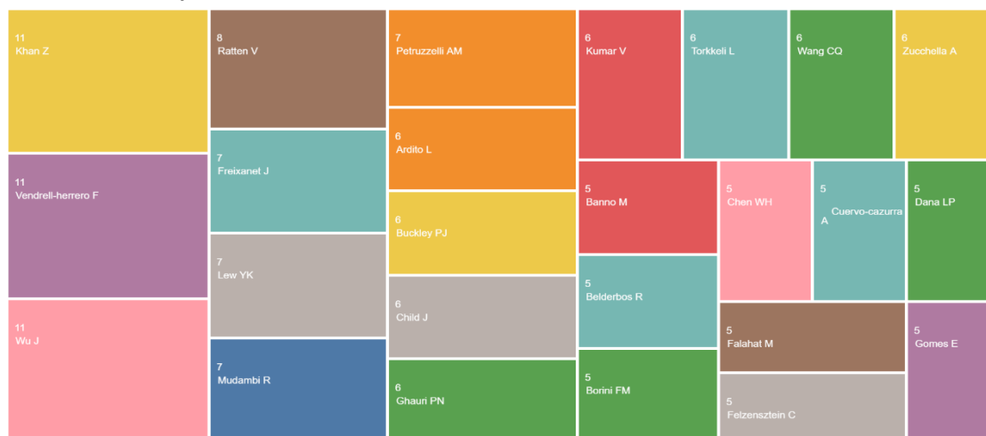
Figura 3 – Autores com Maior Volume de Publicações sobre Inovação e Internacionalização
