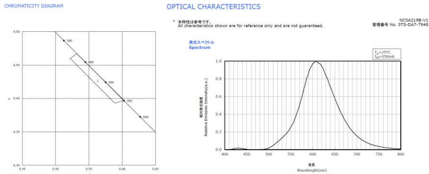
Figura 8: Espectro no diodo fosforo converter blue die FONTE: Nichia Corporate 2018
