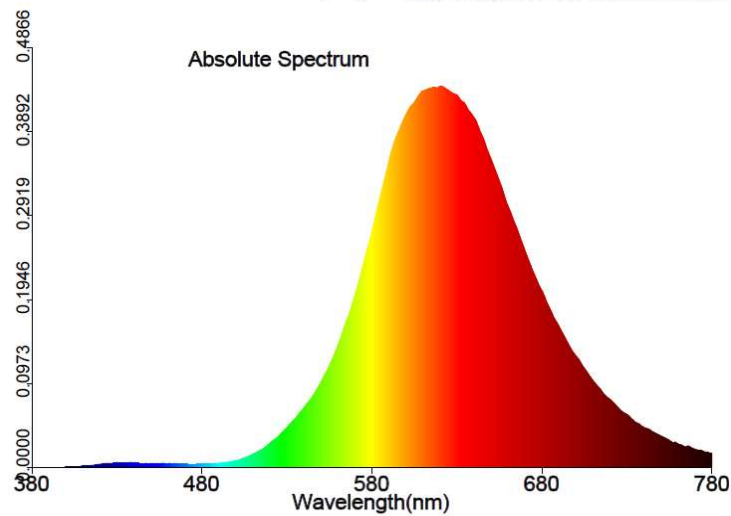
Figura 9: Espectro no novo produto a 605nm Fonte Interlight Iluminação 2018
