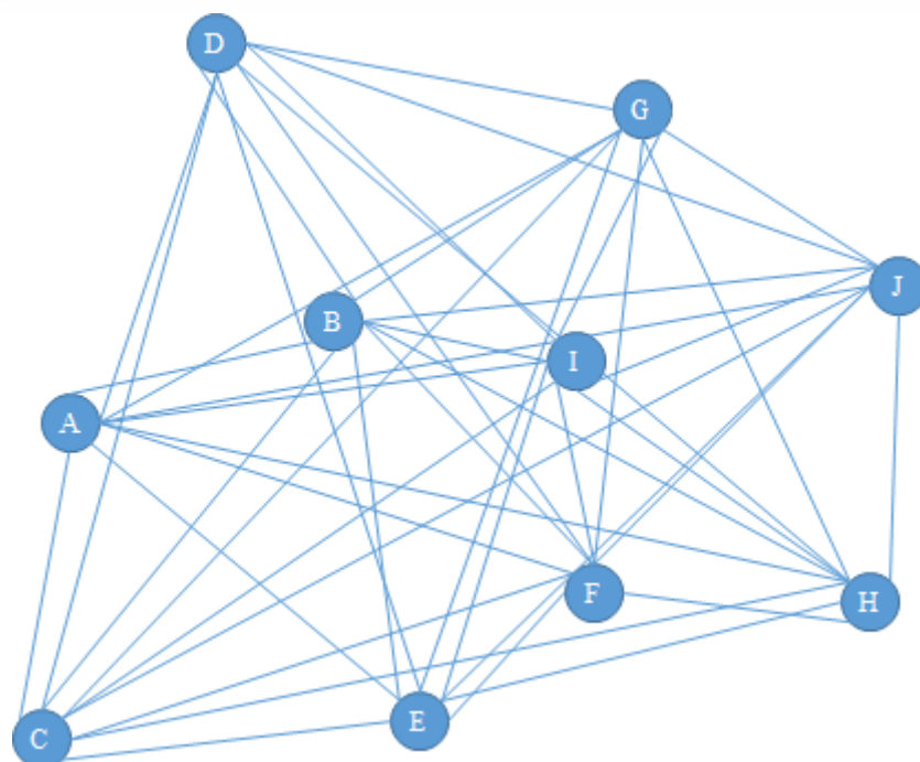
Figura 2. Representação de Grafo
