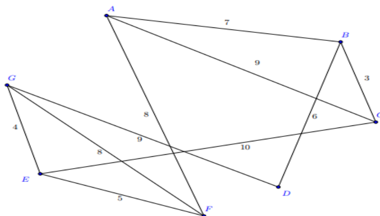
Figura 1. Exemplo de um grafo
