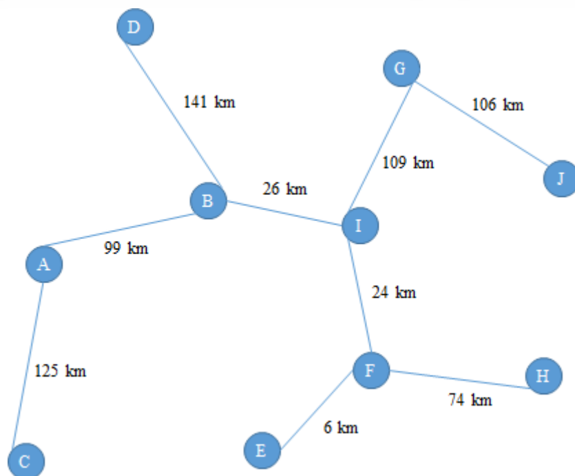
Figura 5. Árvore mínima desenvolvida pelo Algoritmo de Kruskal
