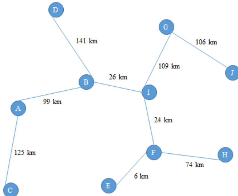
Figura 7. Árvore mínima desenvolvida pelo Algoritmo de Prim
